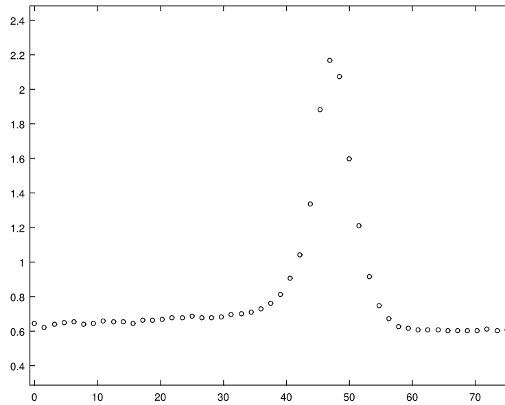
Fig. 5. Titanium heat data (De Boor and Rice, 1968).
